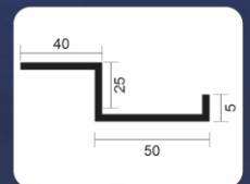
Talang Rembes Tipe L
