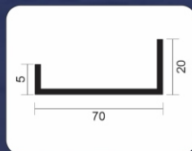
Lisplang Tipe L
